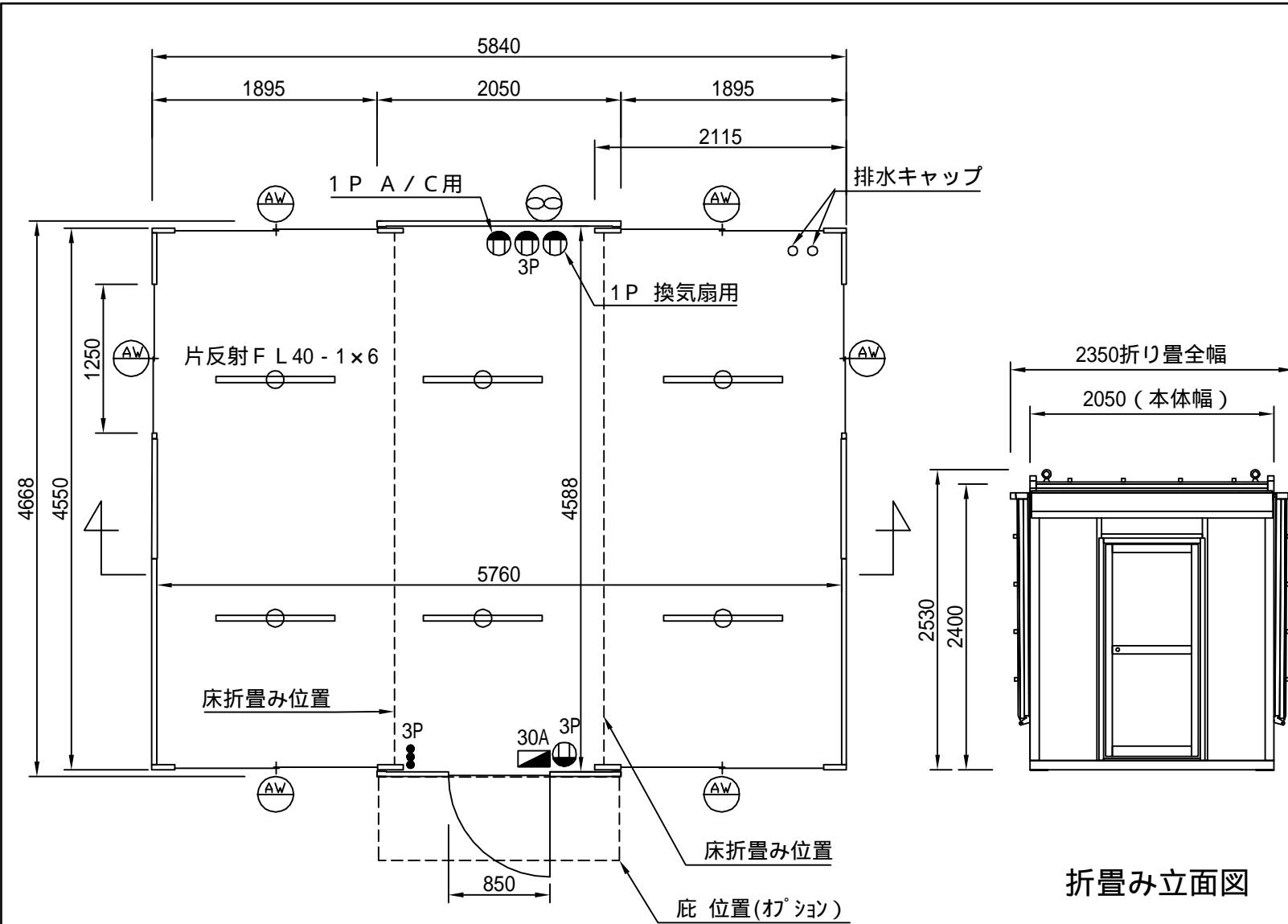
平面図
