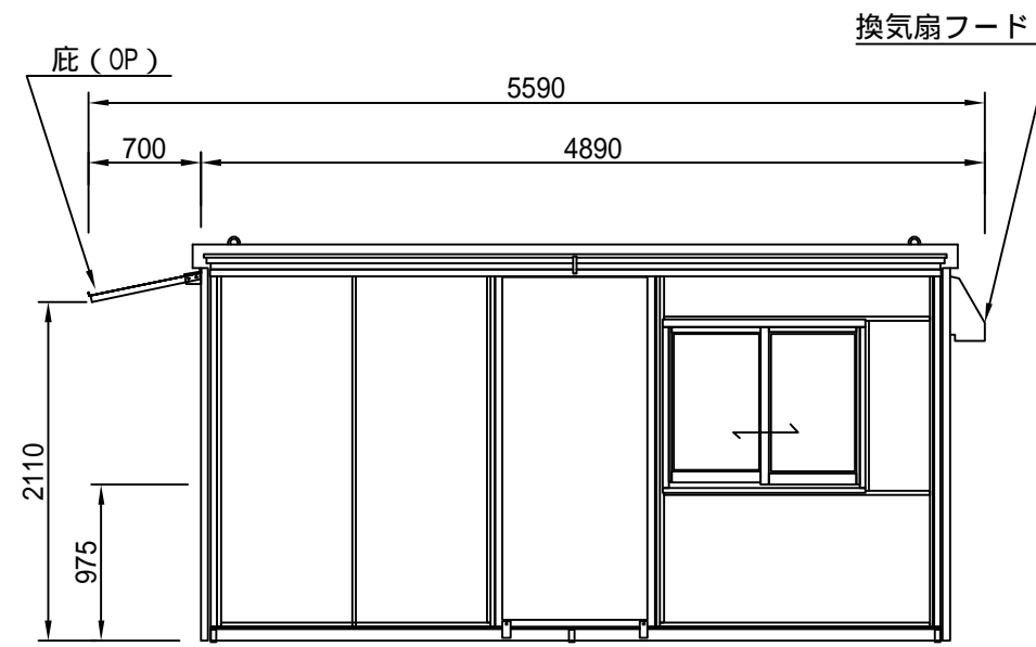
立面図
