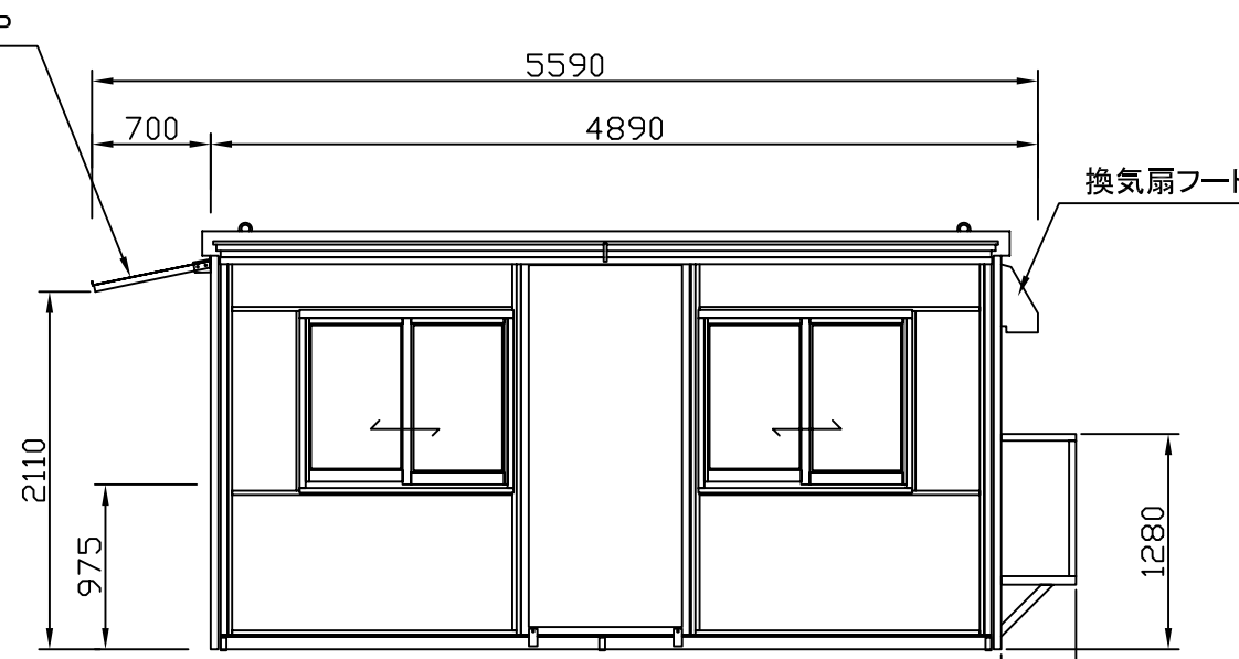
立面図
