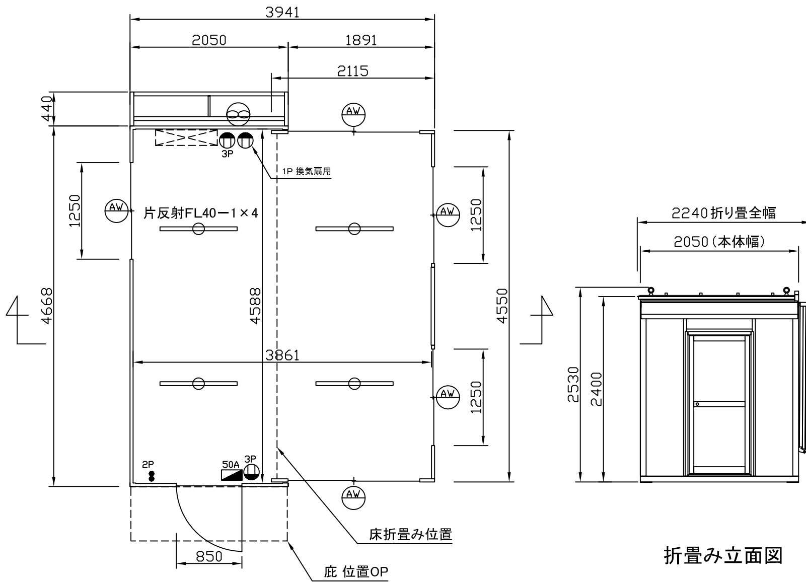
平面図
