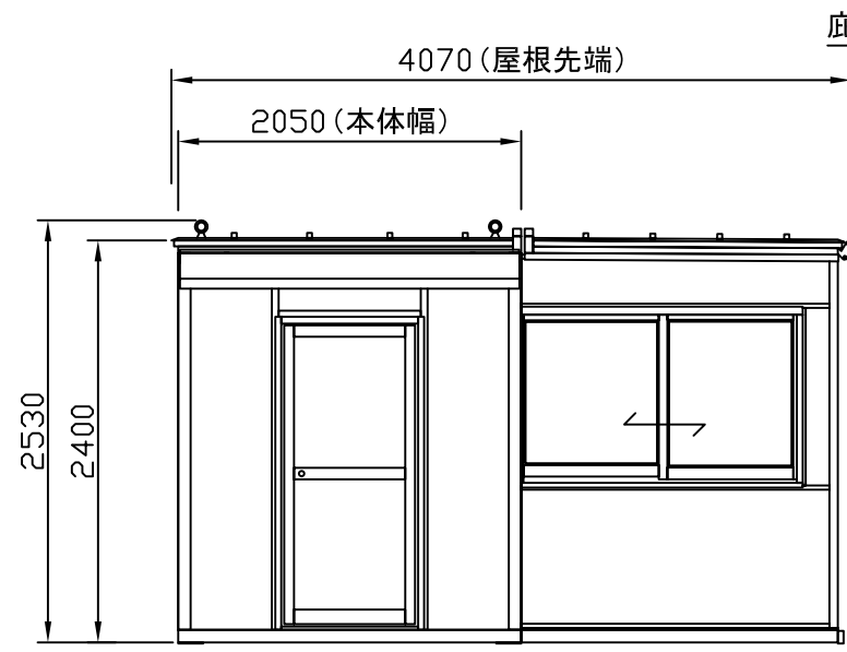
立面図
