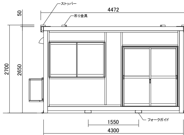
C面立面図
