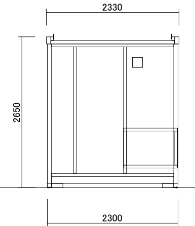
D面立面図
