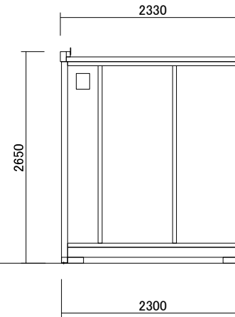
B面立面図
