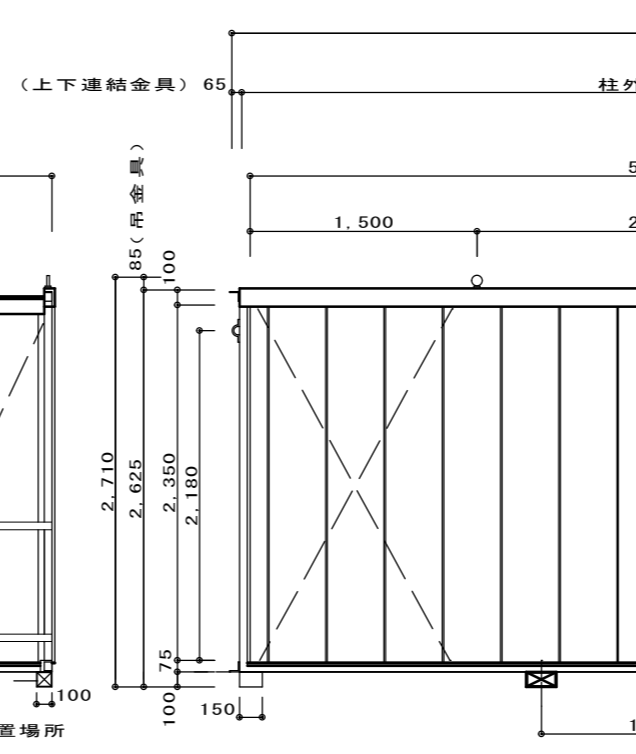
C面立面図
