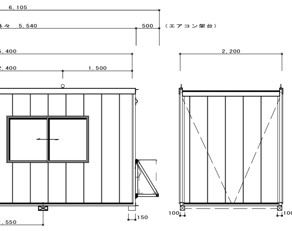
D面立面図
