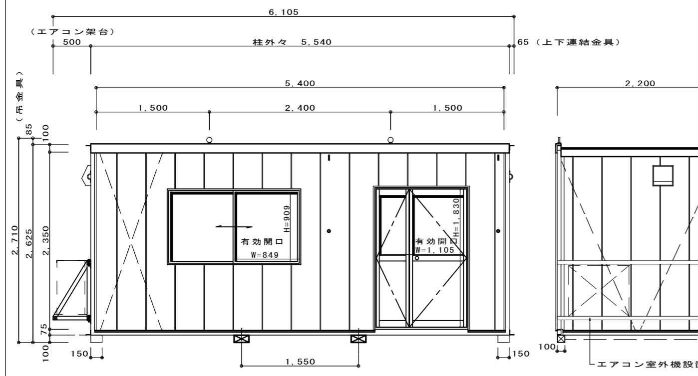
A面立面図
