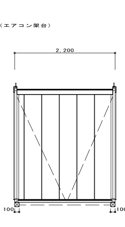
D面立面図
