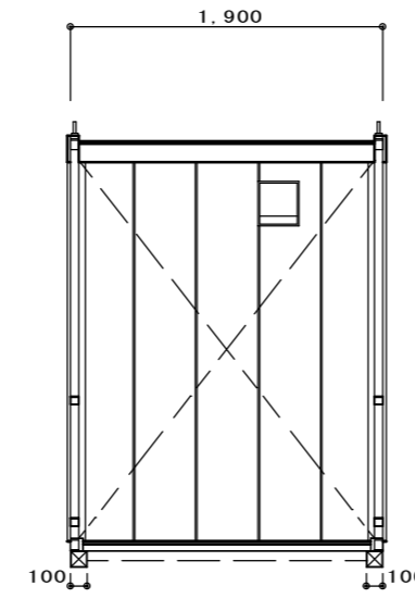
B面立面図
