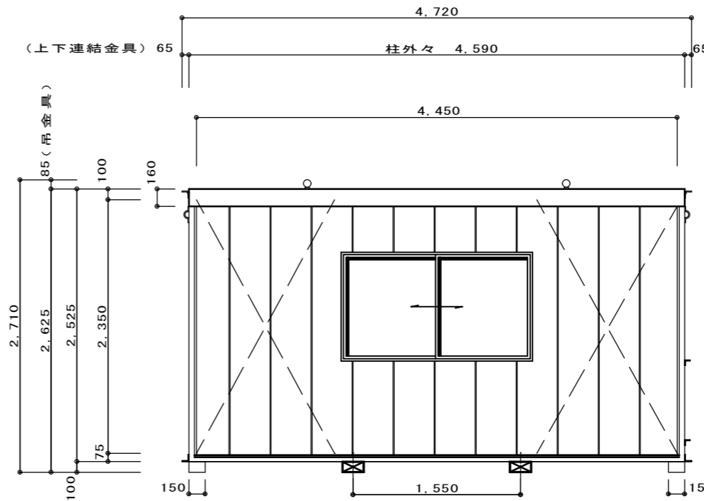
C面立面図
