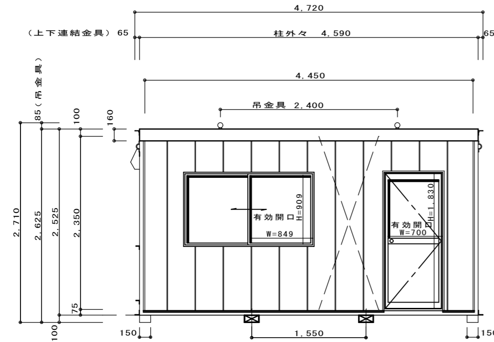
A面立面図
